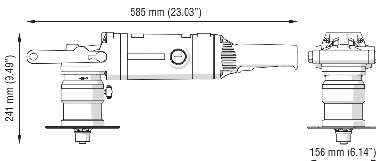
Obaranje ivica sa radijusom
