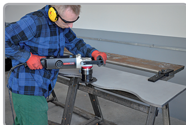
Obaranje zakrivljenih ivica
